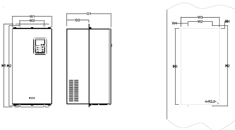
Рисунок В-10 Фланцевый монтаж для моделей 37 – 110 кВт (G-тип)
