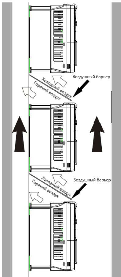
Рис. 4-5 Вертикальная установка
