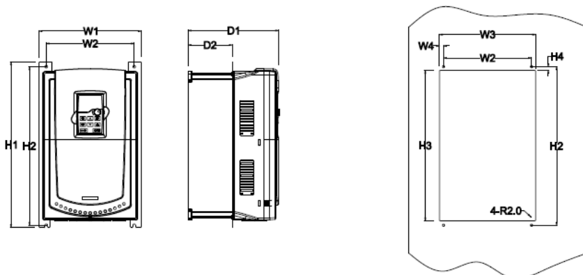
Рисунок В-9 Фланцевый монтаж для моделей 18 – 30 кВт (G-тип)
