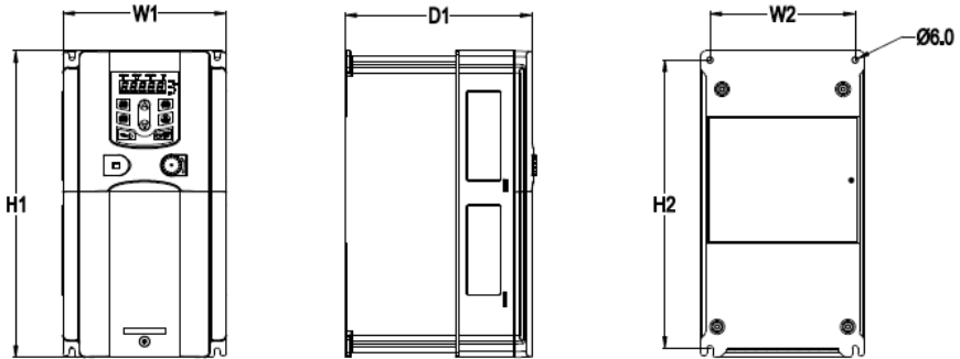
Рисунок В-3 Настенный монтаж для моделей 0,75 – 15 кВт (G-тип)
