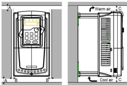
Рис. 4-3 Одиночная установка
